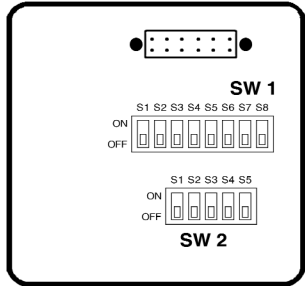
Ansicht Rückseite
